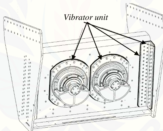
Gambar 2.10 Vibrator Unit (Metso, 2016)
