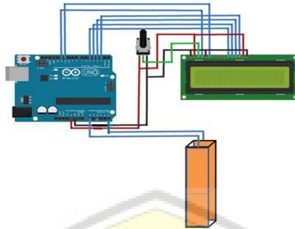
Gambar 2. Rangkaian Alat Ukur Curah Hujan
