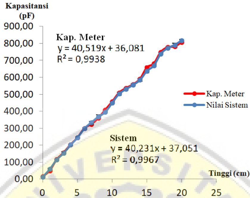
Gambar 4. Hubungan tinggi level air dengan kapasitansi
