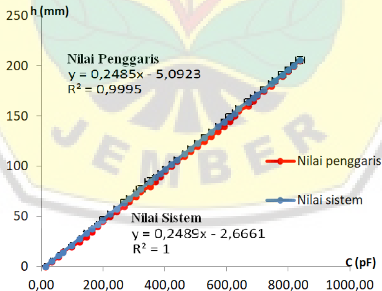
Gambar 5. Hubungan nilai kapasitansi dan tinggi air melalui pembacaan dari sistem dan penggaris
