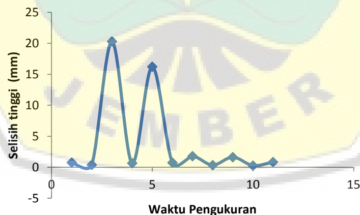
Gambar 6. Grafik hubungan selisih curah hujan yang terukur antara kedua alat dengan waktu pengukuran
