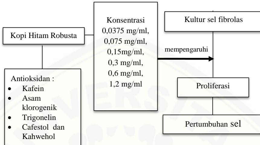
Gambar 2.6 Kerangka Konseptual
