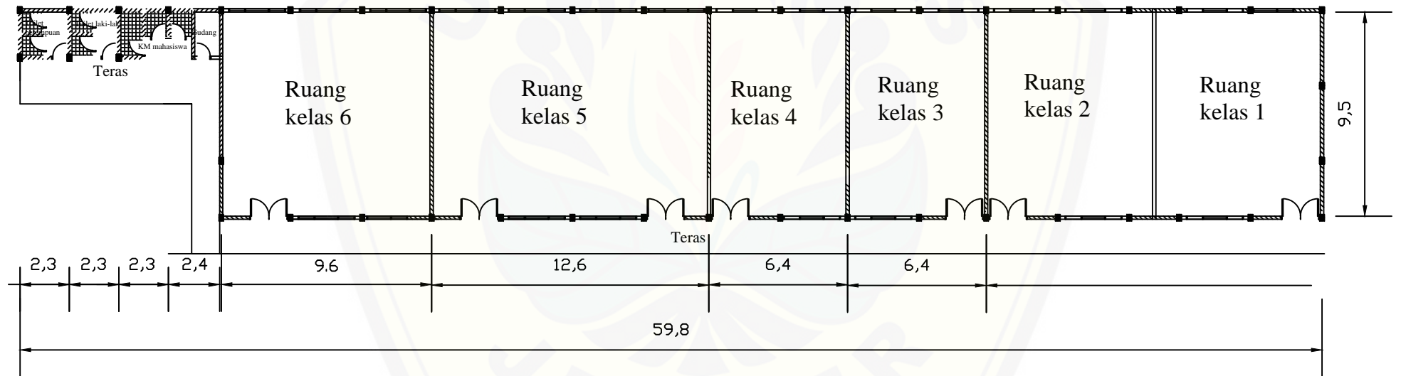
Denah Gedung Ruang kelas Skala 1:250
