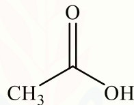
Gambar 2.15 Struktur asam asetat (Sumber: Rowe dkk., 2009)
