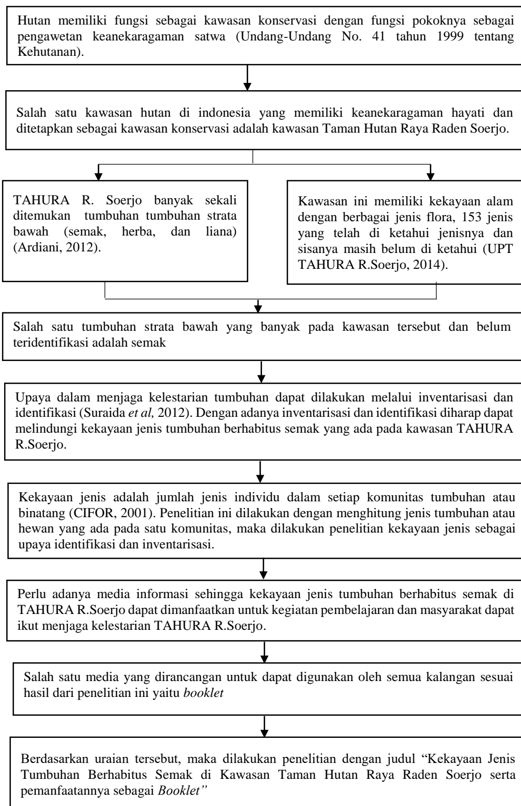
Gambar 2. 1 Kerangka Konseptual
