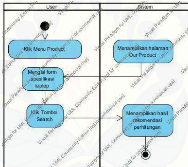
Gambar 4.1 Activity Diagram Melihat Hasil Rekomendasi Laptop
