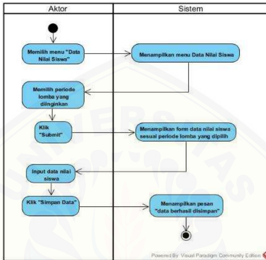
Gambar 8. Activity Diagram Pengelolaan Data Nilai Siswa
