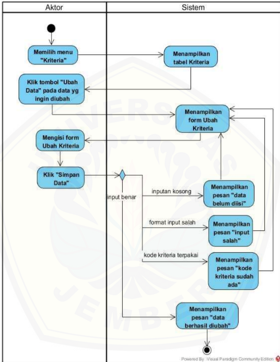
Gambar 10. Activity Diagram Pengelolaan Data Kriteria (Ubah Data)
