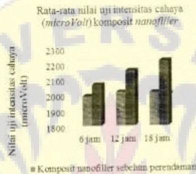
Gambar 1. Histogram rata-rata nilai uji intensitas cahaya (microVolt) komposit nanofiller
