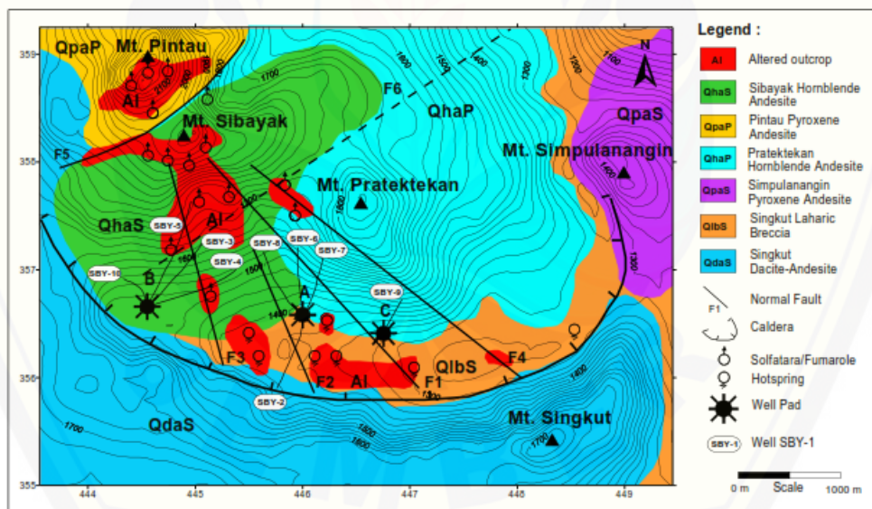
Gambar 2.1 Peta Geologi Lapangan Geotermal Daerah Sibayak (Daud, 2000).
