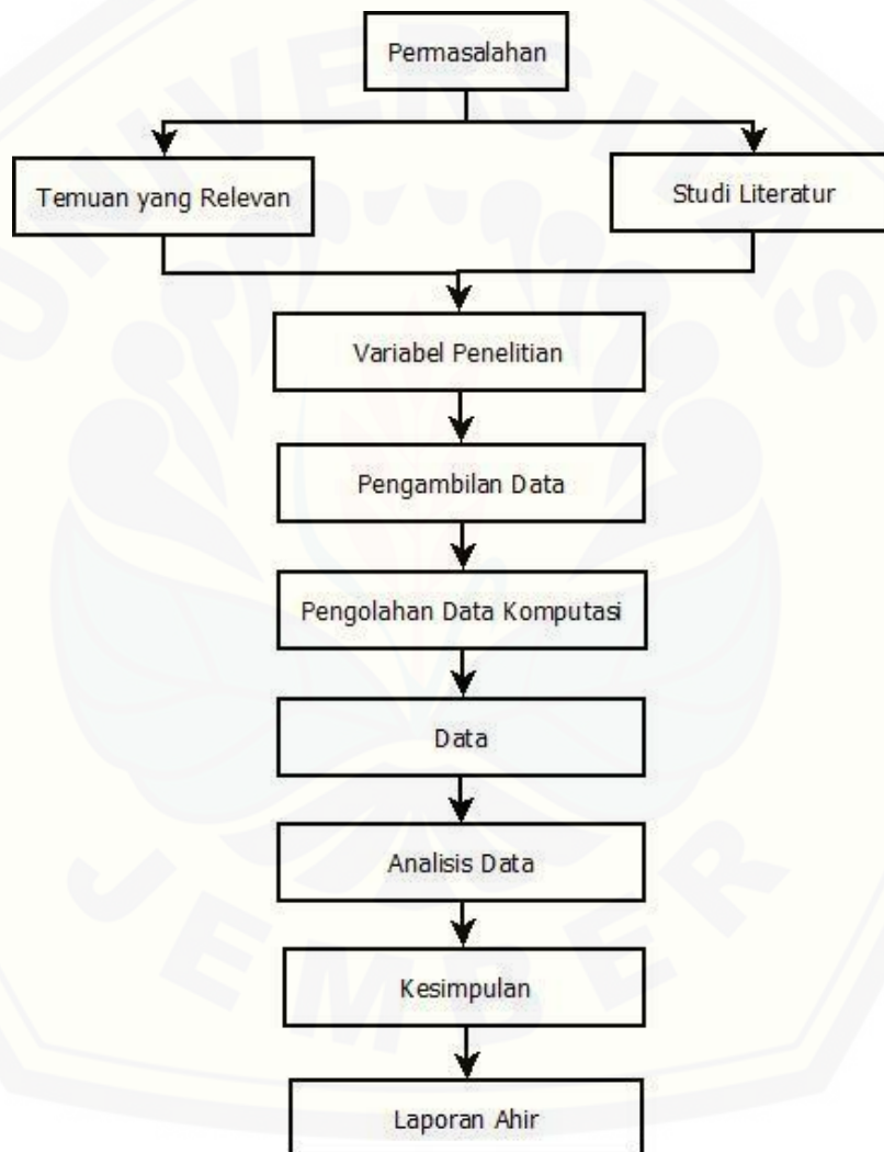
Gambar 3.1 Rancangan Penelitian
