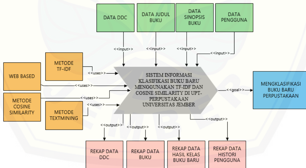
Gambar 4.1 Bisnis Proses Sistem Informasi Klasifikasi Buku Perpustakaan
