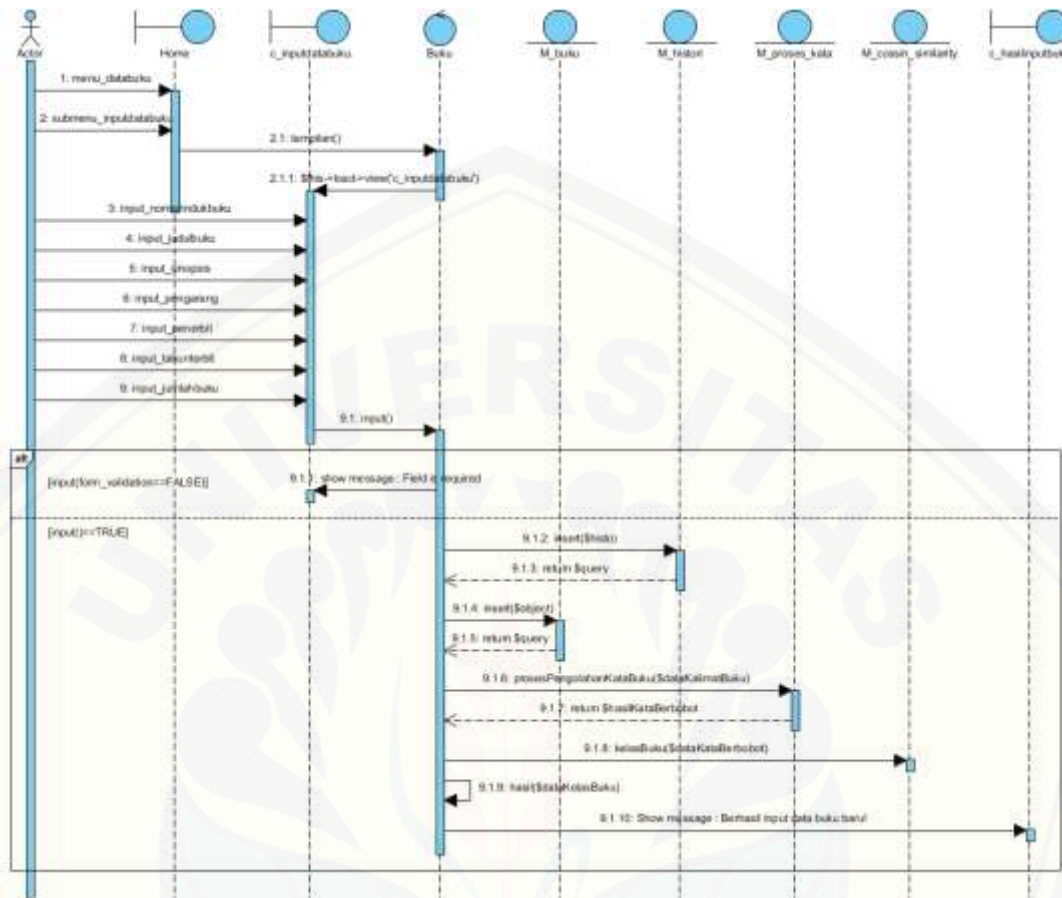
Gambar 4.12 Sequence Diagram Mengelola Data Buku (input)
