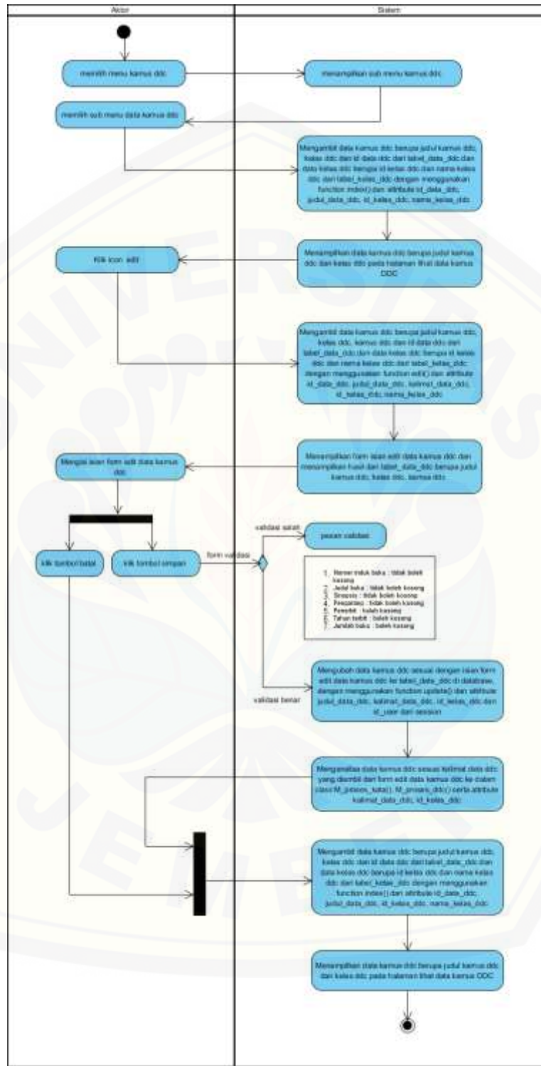
Gambar 4.8 Activity Diagram Mengelola Data Kamus DDC (edit)
