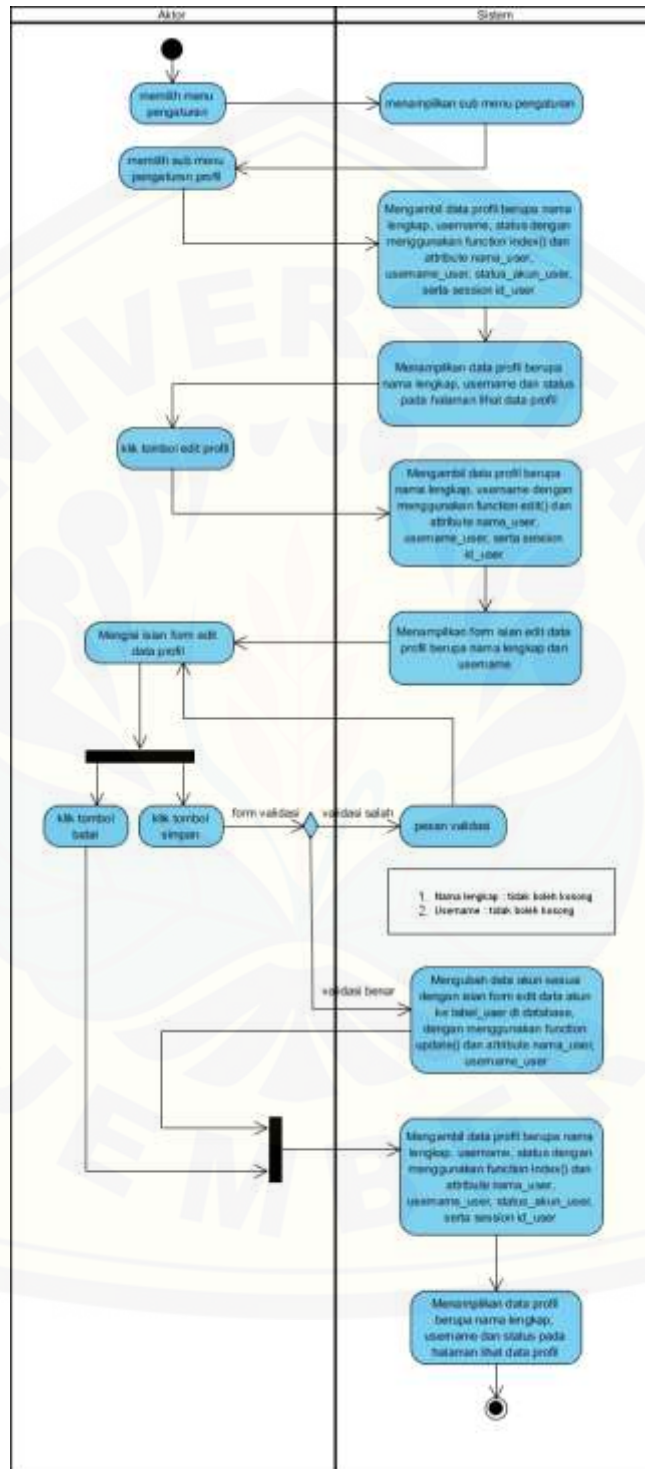
Gambar B.6 Activity Diagram Mengatur Profil ( edit profil )
