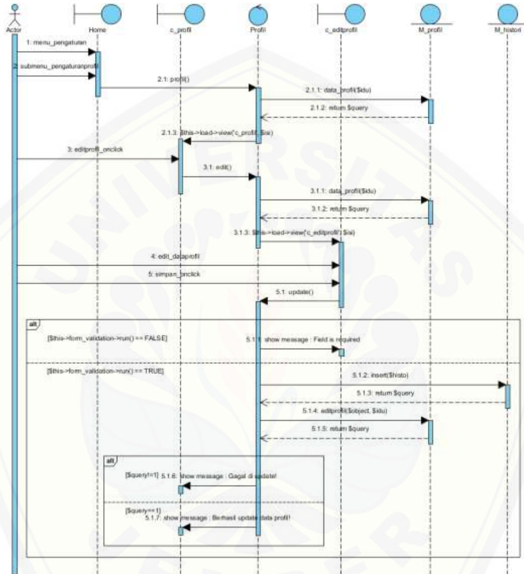
Gambar C.6 Sequence Diagram Mengatur Profil ( edit profil )
