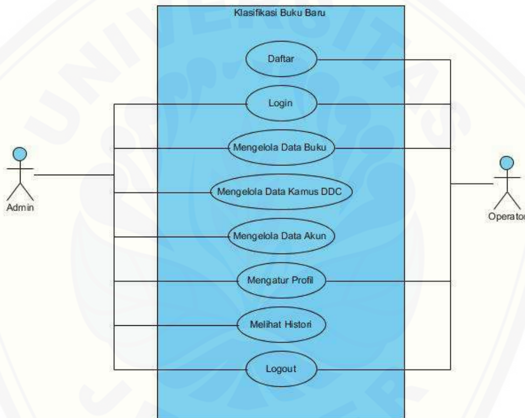
Gambar 4.2 Usecase Diagram Sistem Informasi Klasifikasi Buku Perpustakaan
