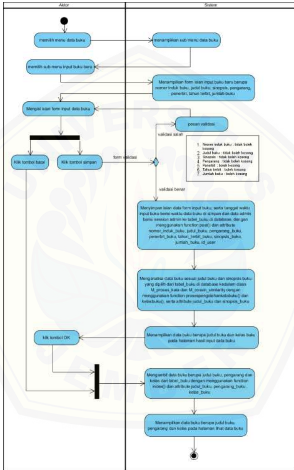
Gambar 4.3 Activity Diagram Mengelola Data Buku (input)
