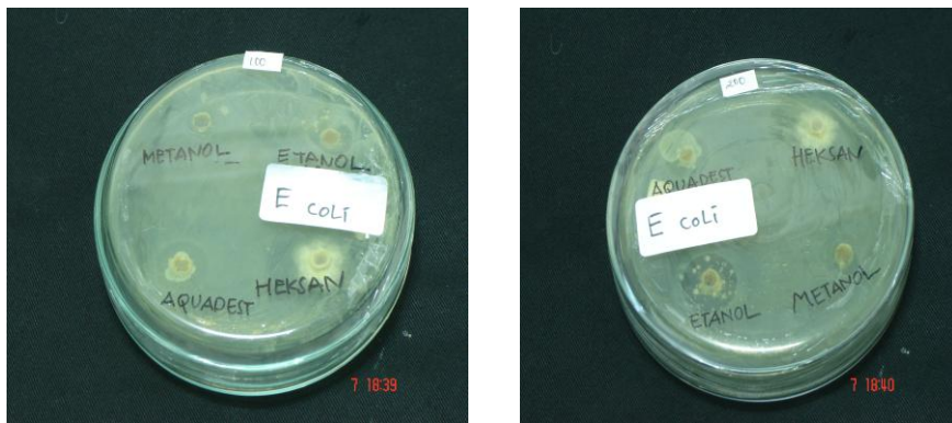
Gambar 9 dan 10. Penghambatan ekstrak benalu konsentrasi 100uL (9) dan 200uL (10) terhadap pertumbuhan Escherichia coli
