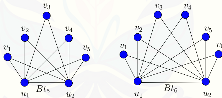
Gambar 2.8 Graf buku segitiga Bt_5 dan Bt_6
