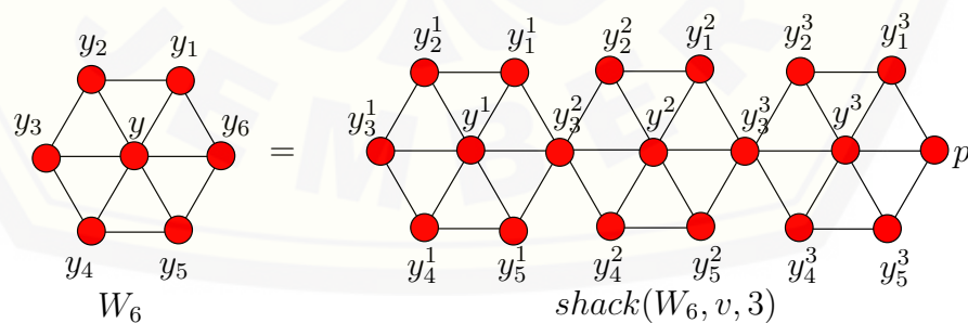
Gambar 2.12 Graf Hasil Operasi Shackle dari W_6
