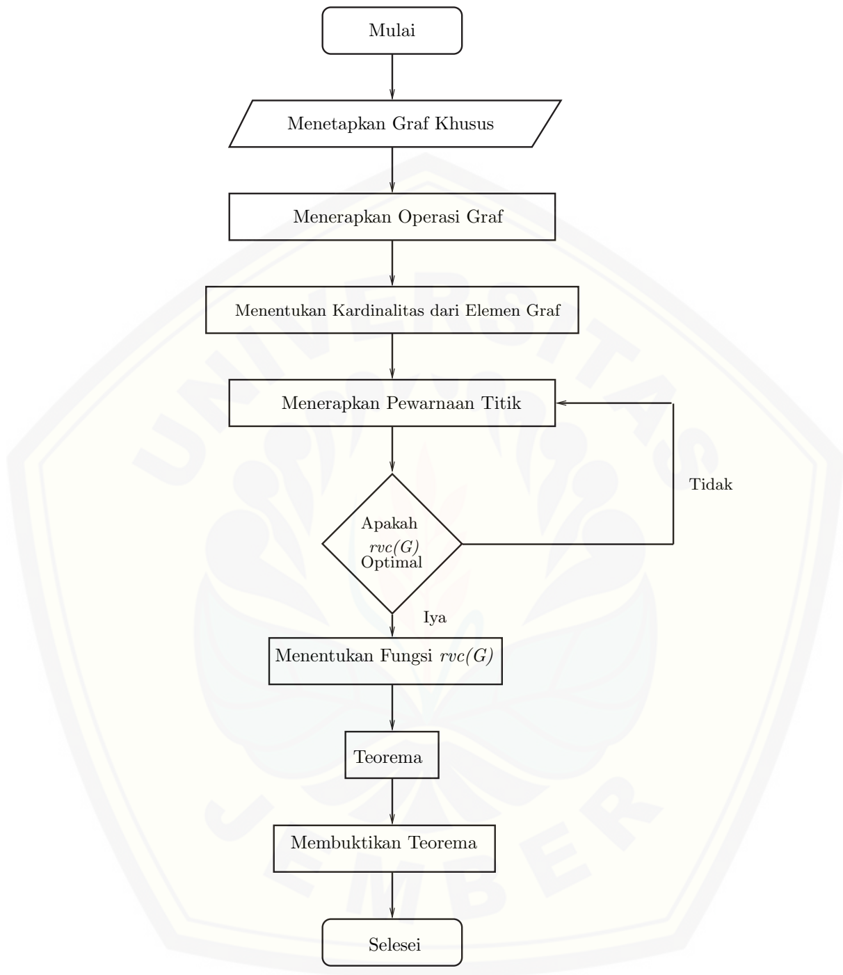
Gambar 3.1 Skema Penelitian
