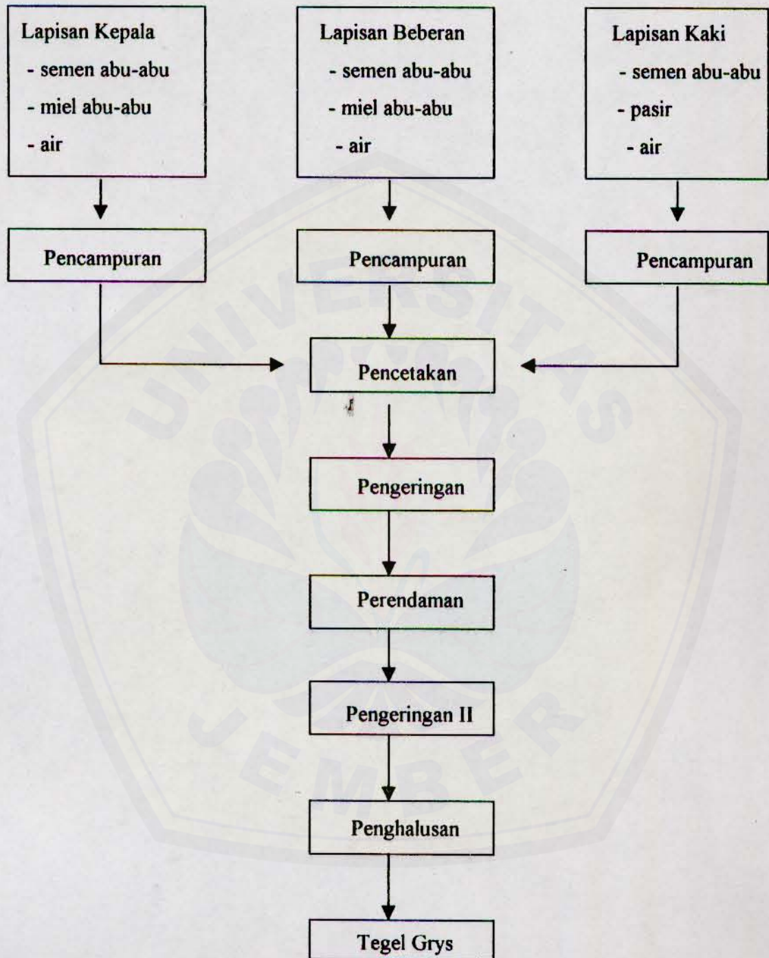
Gambar 3. Skema Proses Produksi Tegel Gry
