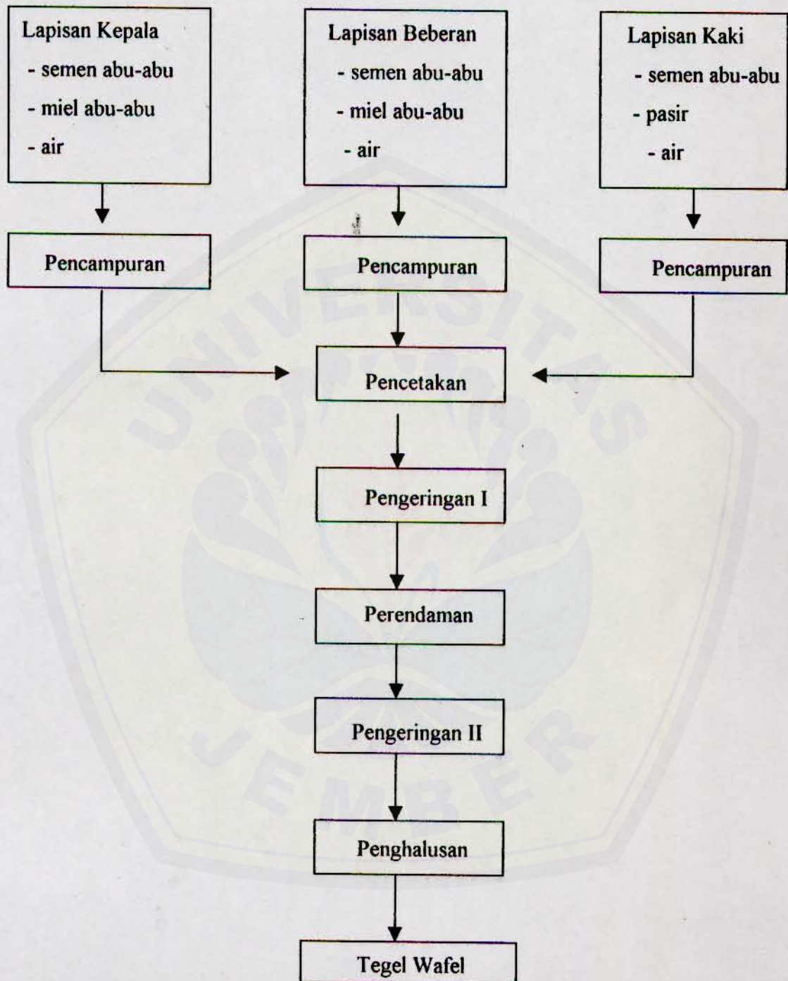
Gambar 5. Skema Proses Produksi Tegel Wafel
