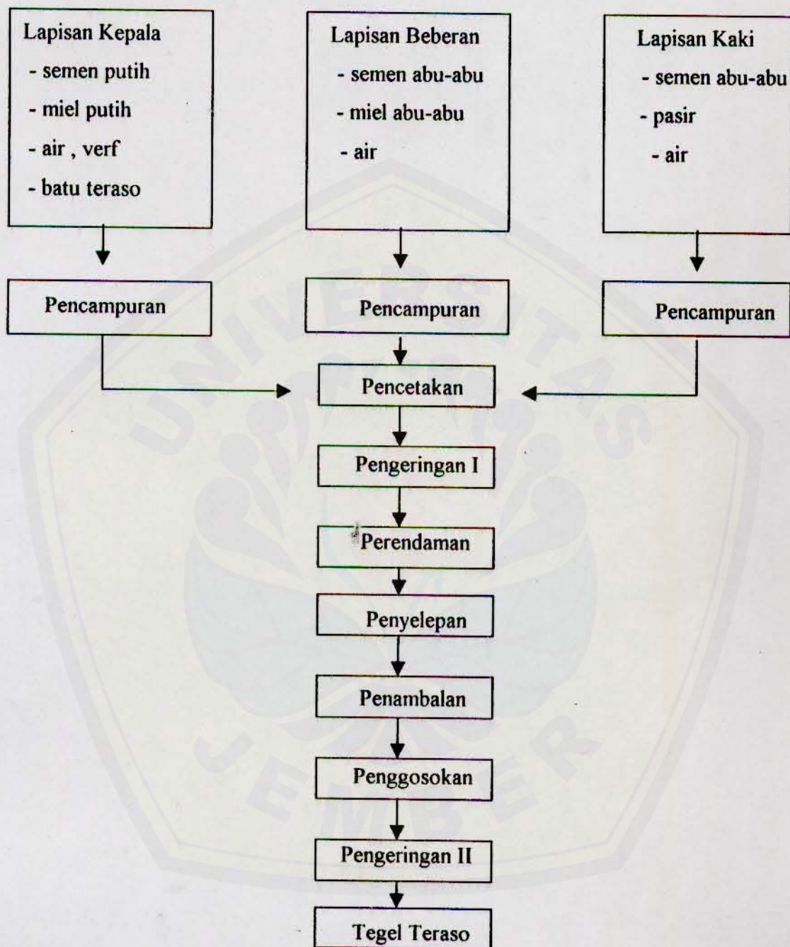
Gambar 6. Skema Proses Produksi Tegel Teraso
