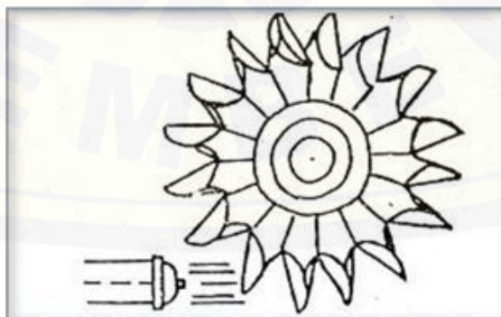
Gambar 2.4 Turbin Aliran Tangensial (Haimerl, L.A., 1960)
