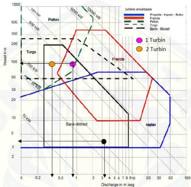
Gambar 4.2 Grafik Pemilihan Turbin
