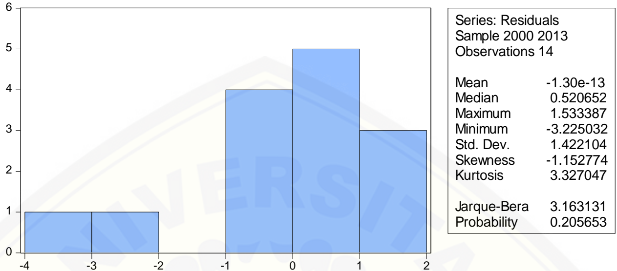
Gambar 4.2 Uji Normalitas
