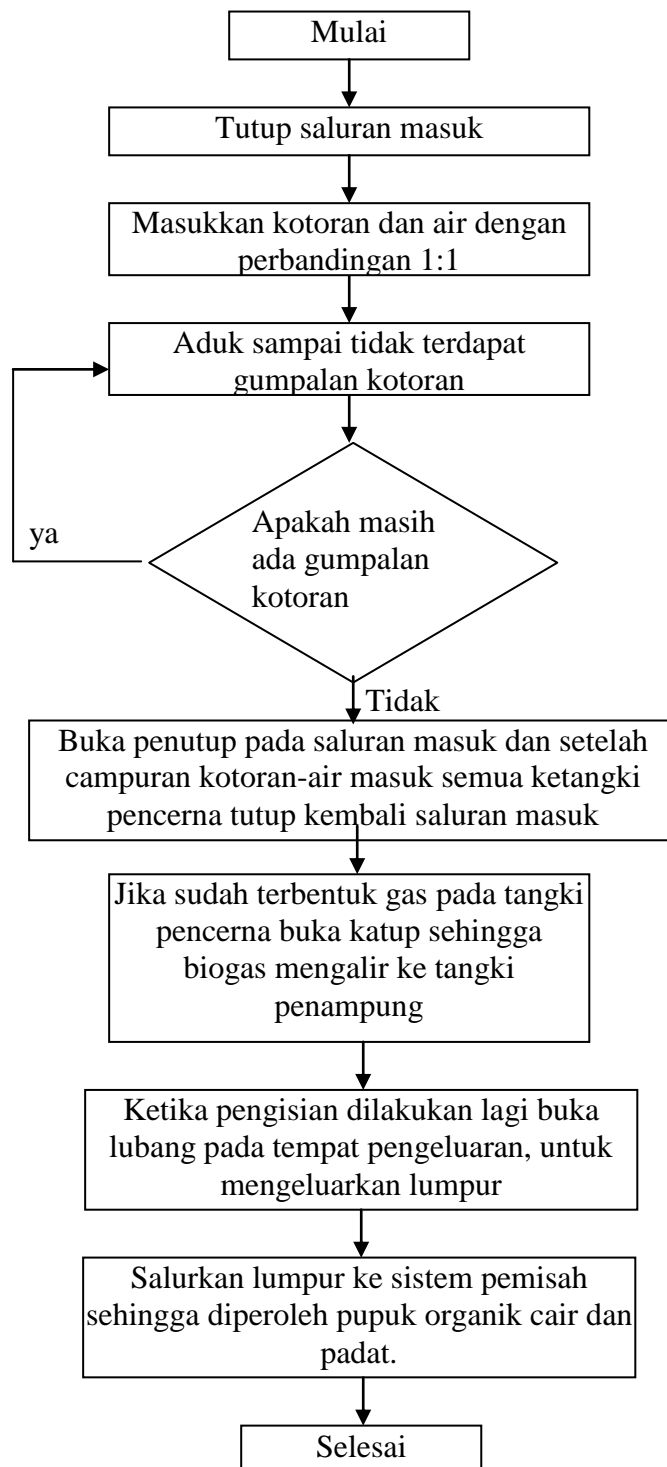
Gambar 2. Cara pengoperasian Sistem Tangki Pencerna Anaerob
