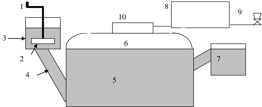
Gambar 1: Sistem Pencerna Anaerobik ( Bioreaktor ) Biogas
