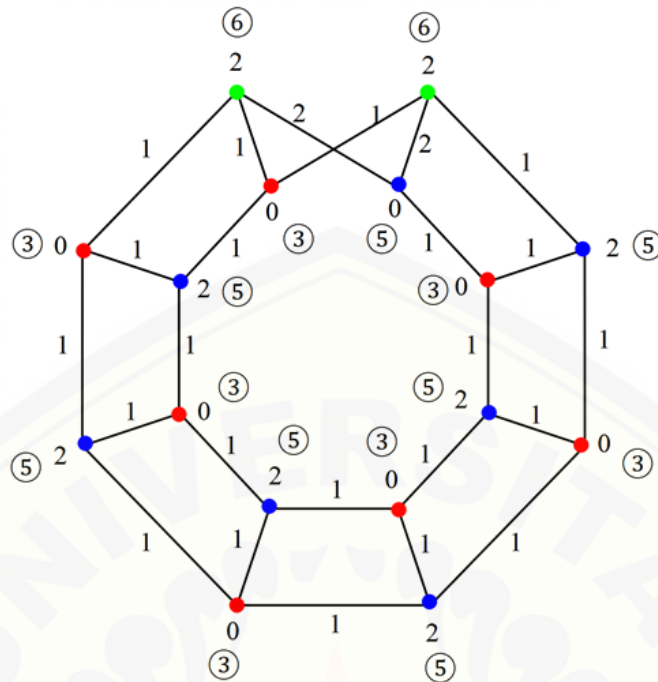
Figure 3. Pewarnaan titik ketakaturan lokal refleksif pada graf tangga möbius ( M_n ) untuk n = 8
