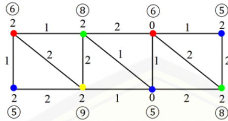
Figure 1. Pewarnaan titik ketakteraturan lokal refleksif pada graf tangga segitiga ( TL_n ) untuk n = 4
