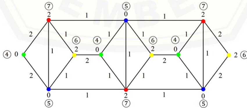
Figure 2. Pewarnaan titik ketakteraturan lokal refleksif pada graf tangga permata ( DL_n ) untuk n = 3
