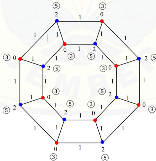
Figure 4. Pewarnaan titik ketakteraturan lokal refleksif pada graf tangga melingkar ( CL_n ) untuk n = 8
