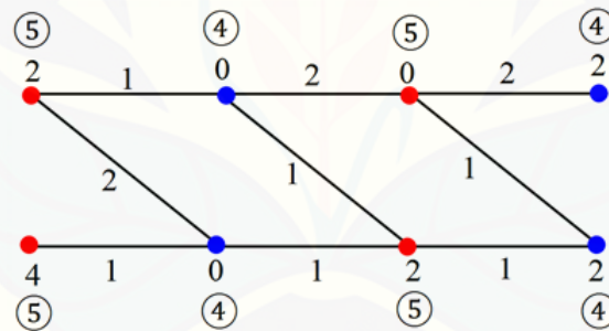
Figure 5. Pewarnaan titik ketakteraturan lokal refleksif pada graf tangga miring ( SL_n ) untuk n = 4
