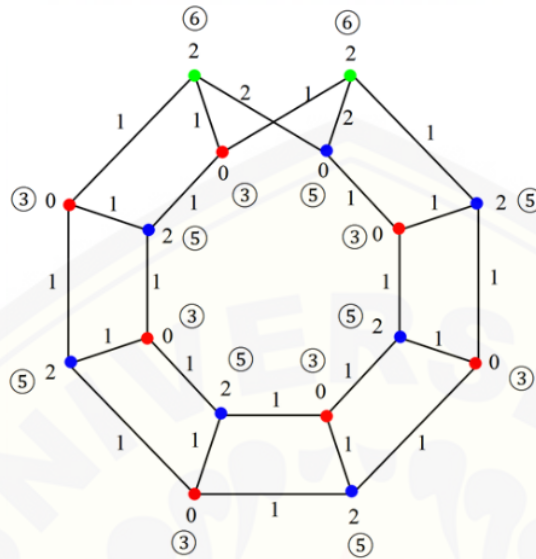
Figure 3. Pewarnaan titik ketakteraturan lokal refleksif pada graf tangga möbius ( M_n ) untuk n = 8
