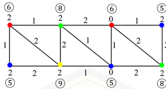
Figure 1. Pewarnaan titik ketakteraturan lokal refleksif pada graf tangga segitiga ( TL_n ) untuk n = 4
