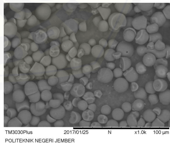
Gambar 1. Hasil Pengamatan Pati Singkong Kuning dan RS Tipe 3 Singkong Kuning dengan SEM dengan perbesaran 1000x.
