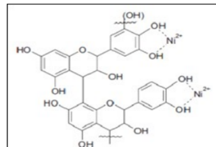
Gambar 2. Reaksi tanin dan ion nikel membentuk lapisan pasif
