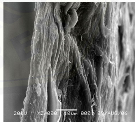
Gambar 10. Hasil SEM membran yang diinkubasi dengan glukosa selama 2 jam (penampang)
