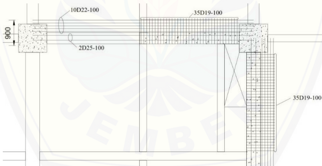
Gambar 7. Penulangan diafragma
