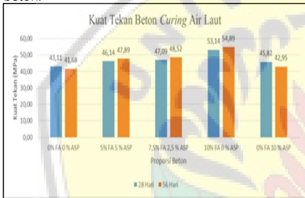
Gambar 6. Perbandingan Kuat Tekan dalam Air Laut
