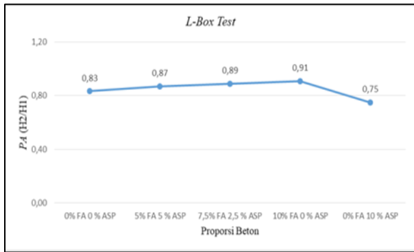
Gambar 3. Grafik Uji L-Shaped Box
