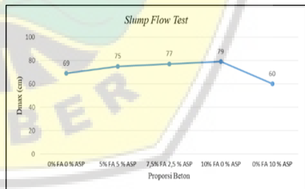
Gambar 2. Grafik Uji Slump Flow
