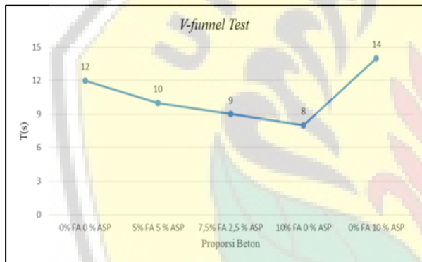
Gambar 4. Grafik Uji V-funnel
