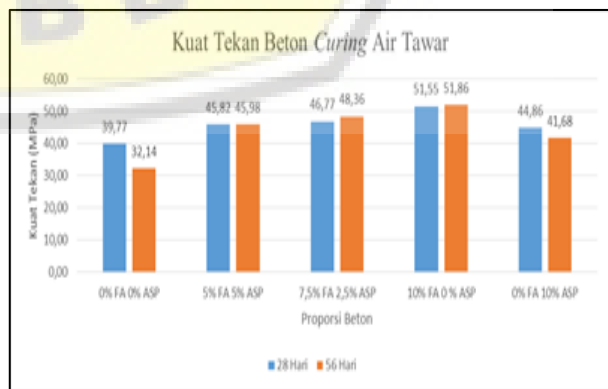
Gambar 5. Perbandingan Kuat Tekan dalam Air Tawar
