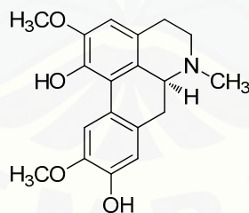
(+)-isoboldine 17
