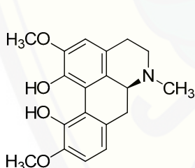
(+)-corytuberine 16
