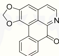
liriodenine 11
