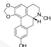
(-)-anolobine 27
