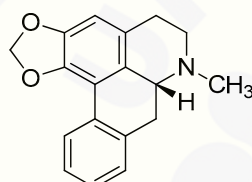
(+)-anonaine 28
