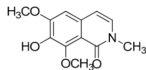
cherianoine 24
