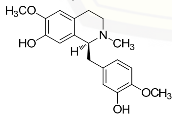
(+)-reticuline 19
