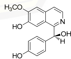
Annocherine A 21
