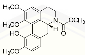
(-)-romucosine H 26
