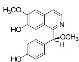
annocherine B 22
