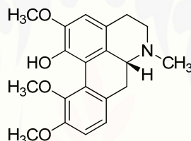
(-)-corydine 29
