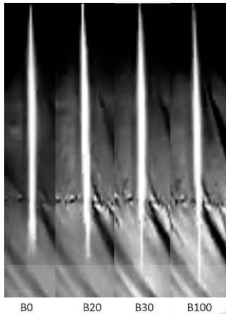
Gambar 3. Karakteristik Spray dengan variasi campuran pada t=6,25 ms
