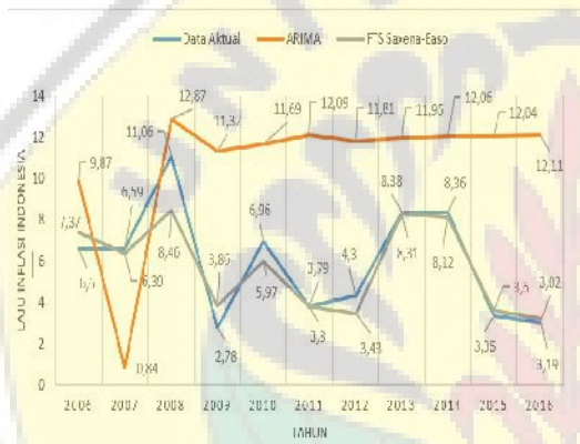
Gambar 2. Perbandingan ketepatan peramalan metode FTS Saxena-Easo dan metode ARIMA terhadap data aktual laju inflasi Indonesia antara periode tahun 2006-2016
