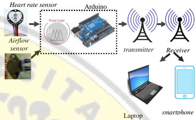
Gambar 7. Skema Perancangan Sistem Telemetry
