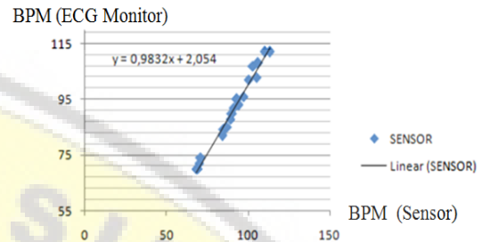
Gambar 17. Kalibrasi Sensor Detak Jantung
