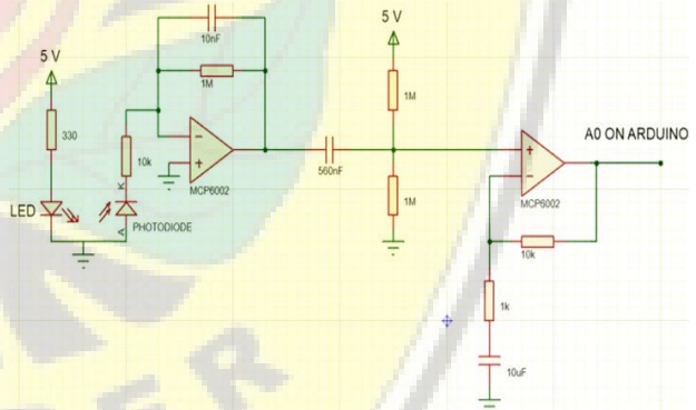
Gambar 3. Rangkaian Sensor Detak Jantung
