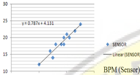
Gambar 18. Kalibrasi Sensor Laju Napas
