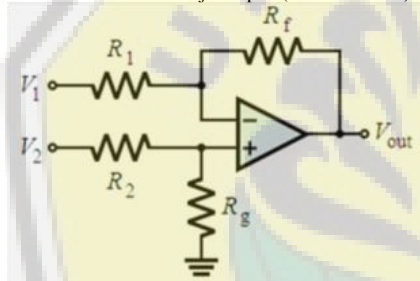
Gambar 5. Rangkaian Penguat Diferensial
