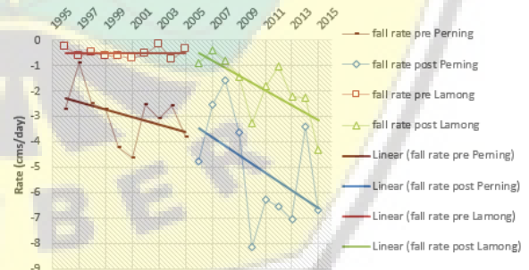
Gambar 19. Penurunan hidrograf
