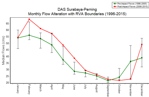
Gambar 4. Perubahan debit bulanan DAS Surabaya Pening
