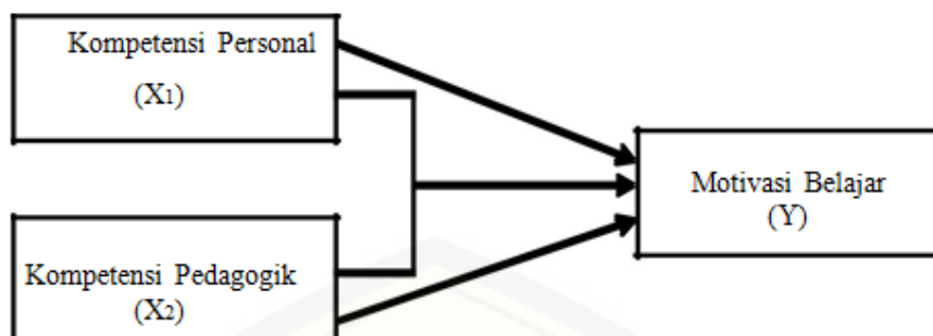
Gambar 3.1 Desain Penelitian
