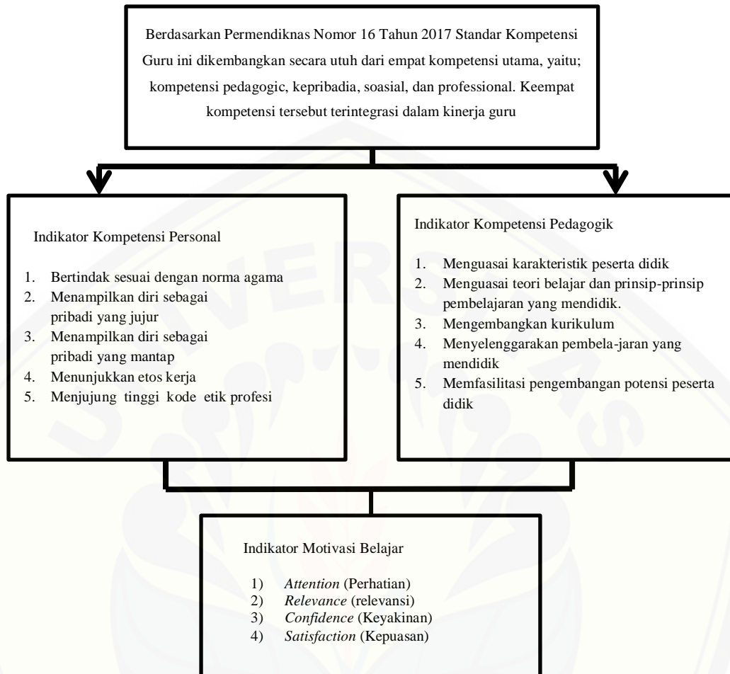
Gambar 2.1 Kerangka Berpikir
