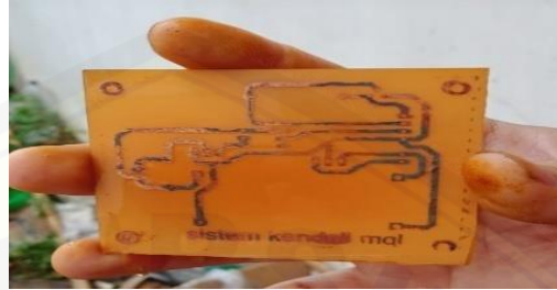
Gambar 3.7 PCB
