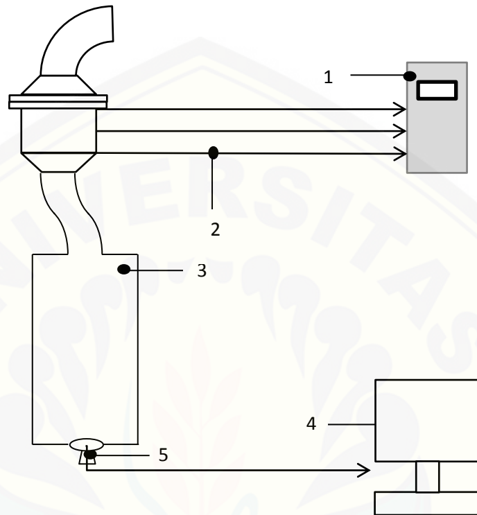
Gambar 3.2 Skema pemasangan alat-alat uji
