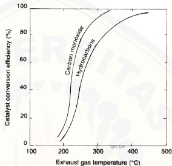
Gambar 2.3 Kurva Efisiensi Konversi Katalis Terhadap Suhu (Sumber: Heisler, 1995)
