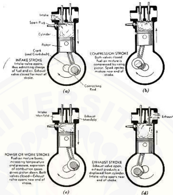
Gambar 2.1 Siklus Motor Bakar 4 Langkah
