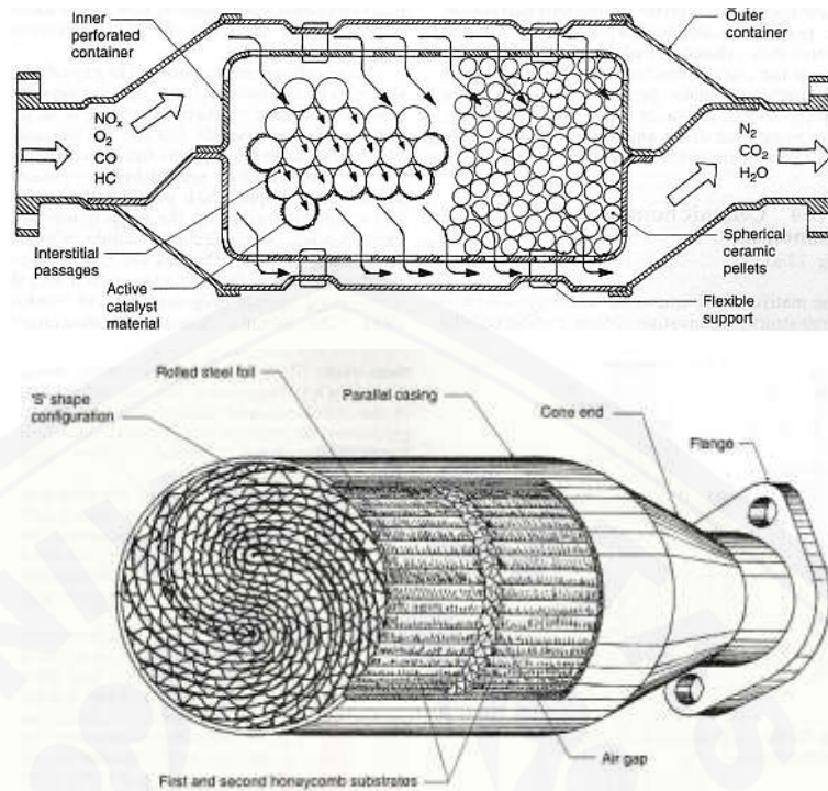
Gambar 2.2 Konstruksi catalytic converter dengan katalis berbentuk butiran (atas) dan monolit (bawah)
