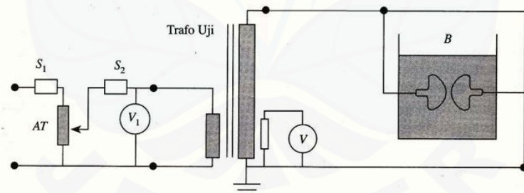
Gambar 14. Rangkaian pengukuran kekuatan dielektrik
