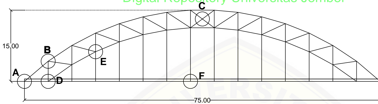
RENCANA BATANG Skala 1 : 400
