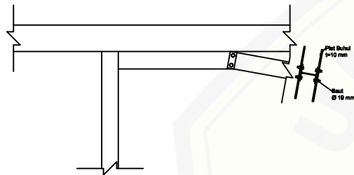
RENC. IKATAN ANGIN LANTAI JEMBATAN Skala 1 : 400
