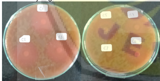
Gambar 1. Diameter zona hambat menunjukkan peningkatan seiring peningkatan konsentrasi vitamin C yg ditambahkan. Keterangan : C1 (klindamisin), C2; C3; C4; C5; C6 (klindamisin + vitamin C 2,5 mg/ml; 5 mg/ml; 10 mg/ml; 20 mg/ml; 40 mg/ml), dan C7 (aquades)
