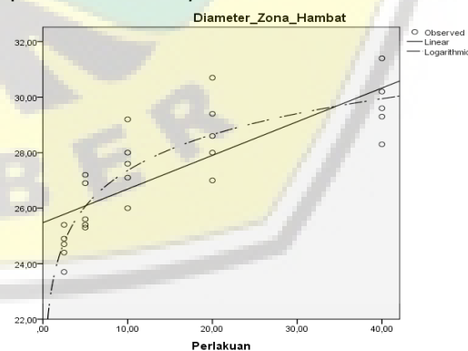
Gambar 2. Kurva konsentrasi vitamin C terhadap diameter zona hambat melalui uji regresi linear dan logaritmik
