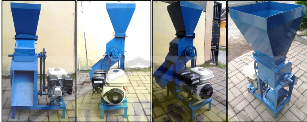
Gambar 10. Mesin pemecah kulit buah kopi
