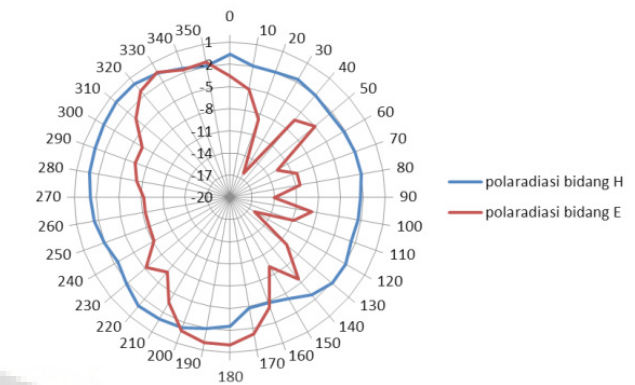
Gambar 26. Pola radiasi antena patch meanderline DGS bidang H dan E
