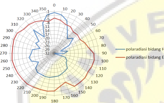
Gambar 24. Pola radiasi antena helix mode axial bidang H dan E
