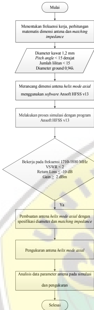
Gambar 3. Diagram alir perancangan antena helix mode axial
