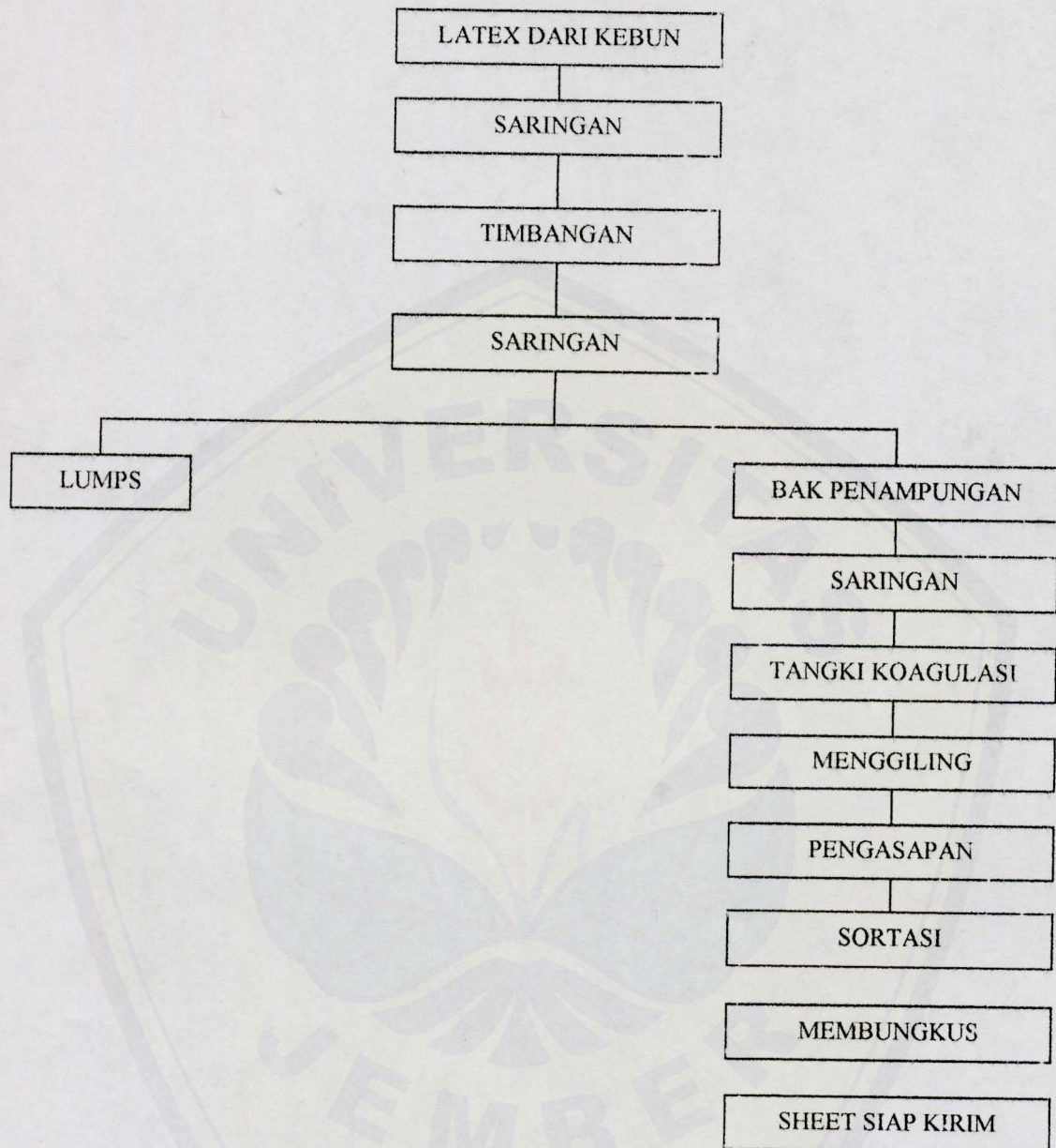
Gambar 3 (tiga) Bagan Pengolahan Karet
