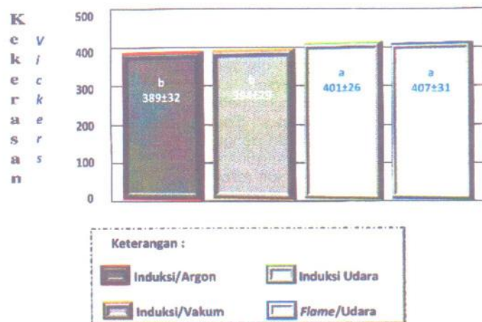
Gambar 5. Rerata kekerasan aloi dengan berbagai metode casting
