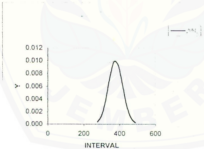
Kurva Distribusi Normal Beton Jenis I
