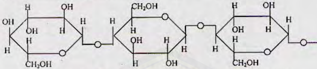
Gambar 2. Struktur Molekul Selulosa (Deman, 1989).
