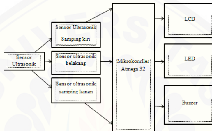
Gambar 2.2 sistem
