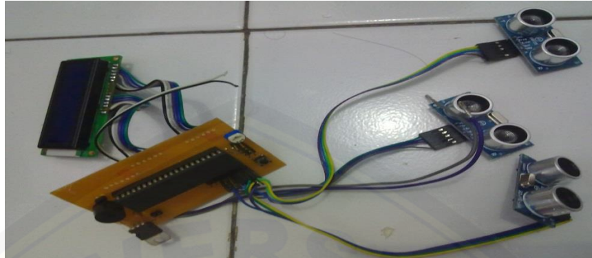
Gambar 2.7 Perancangan Layout
