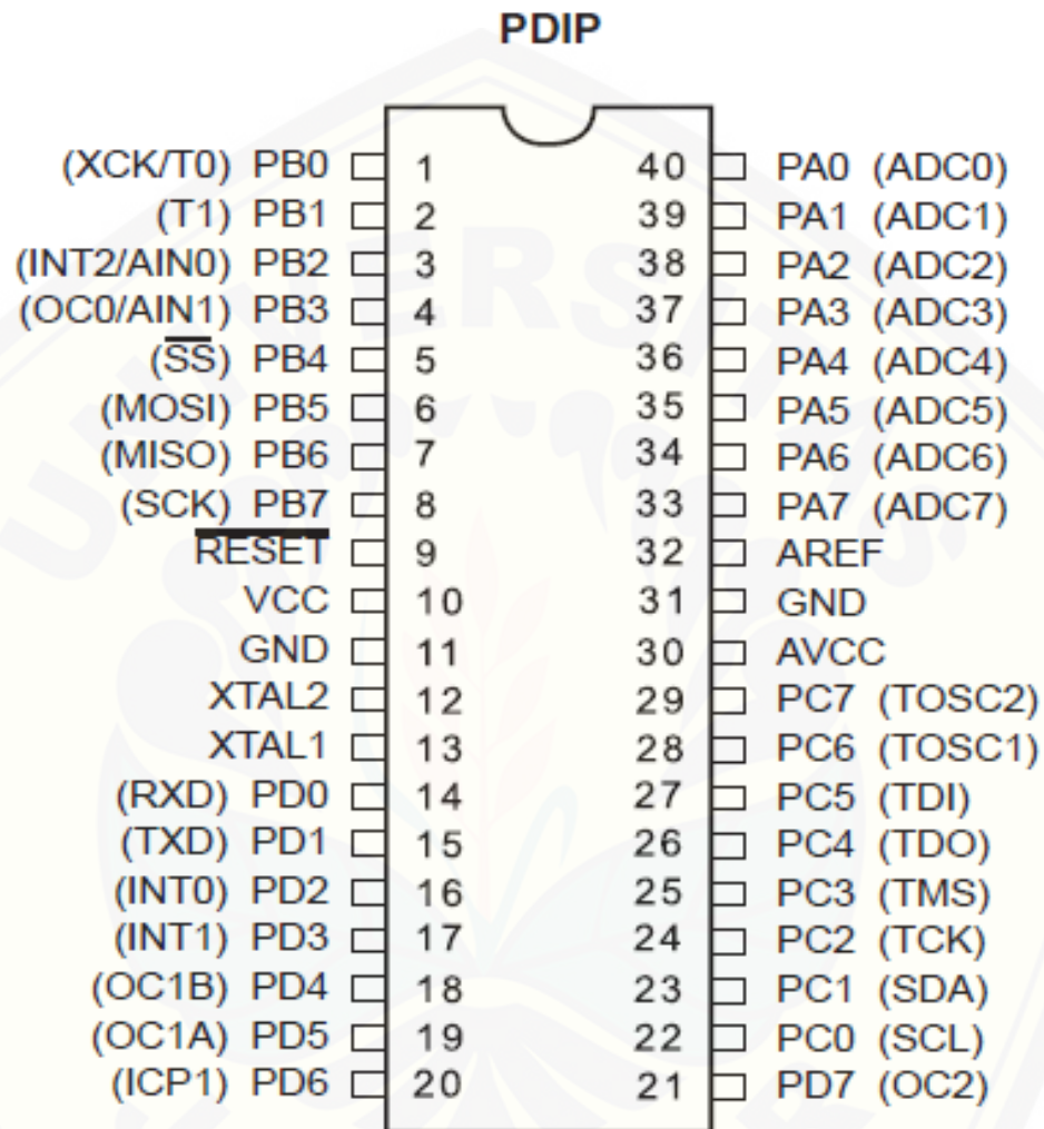
Gambar 1.4 konfigurasi PIN ATmega 32
