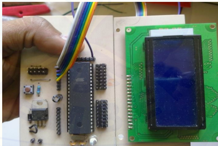
Gambar 3.1 sistem minimum ATmega 32 yang telah dihubungkan dengan LCD
