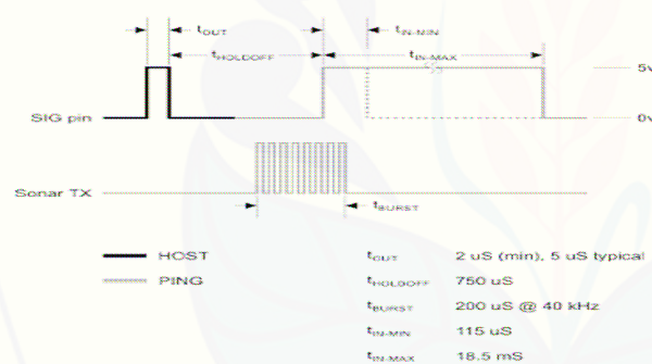
Gambar 6 Siklus Waktu Sensor Ultrasonik
