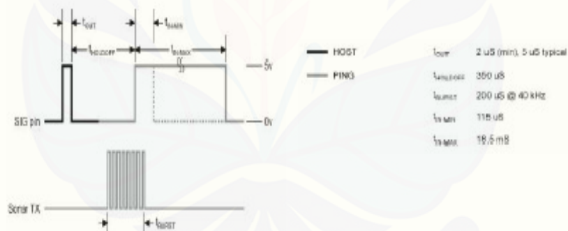
Gambar. 10 Diagram Waktu Sensor
