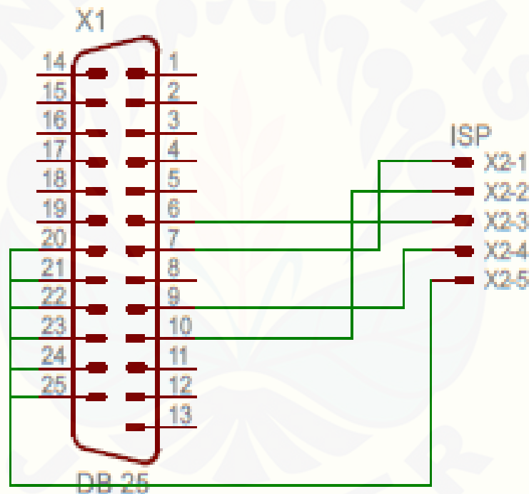
Gambar 3.2 Skema Rangkaian ISP
