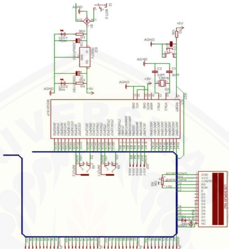
Gambar 3.0 Rangkaian Sistem minimum Dan LCD
