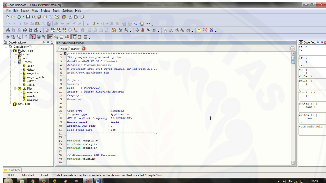
Gambar 1.9 interface codevision-AVR
