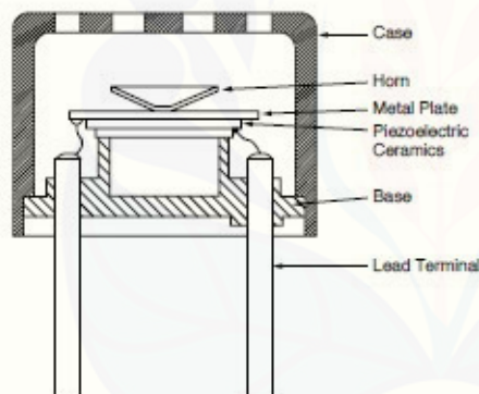
Gambar. 3 konstruksi transduser ultrasonik
