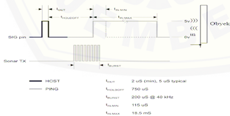
Gambar 5 cara kerja sensor ultrasonik
