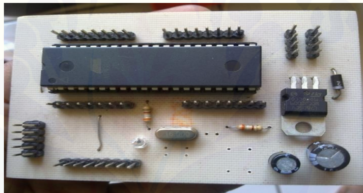
Gambar 2.9 Penempatan komponen
