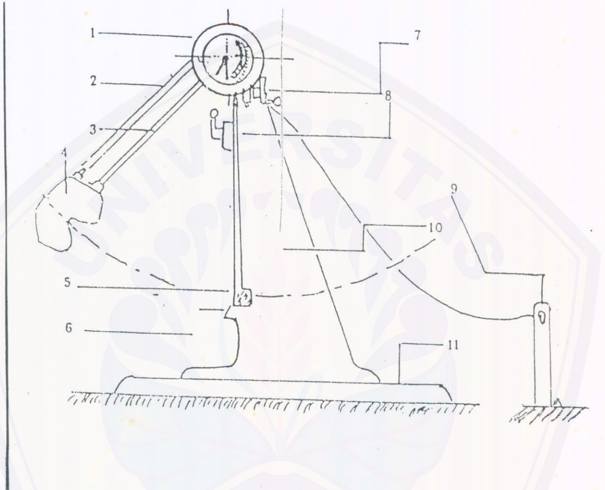
Gambar tes impak Charpy
