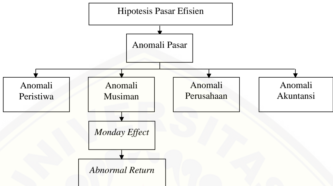
Gambar 2.1 Kerangka Konseptual
