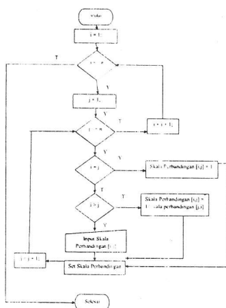
Gambar 2. Pengaturan Skala Perbandingan AHP
