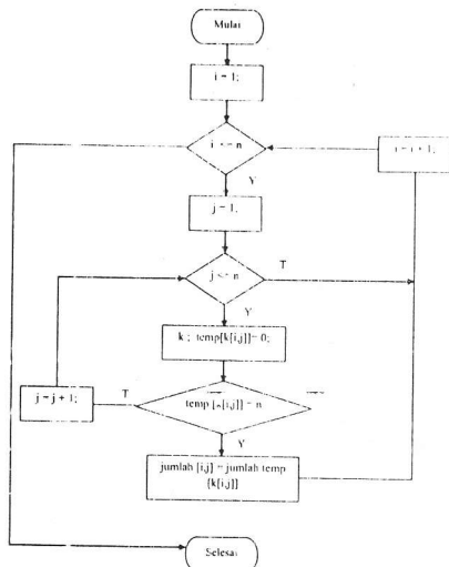
Gambar 5. Penjumlahan Skala Perbandingan Baru Setiap Kriteria Perkolom.
