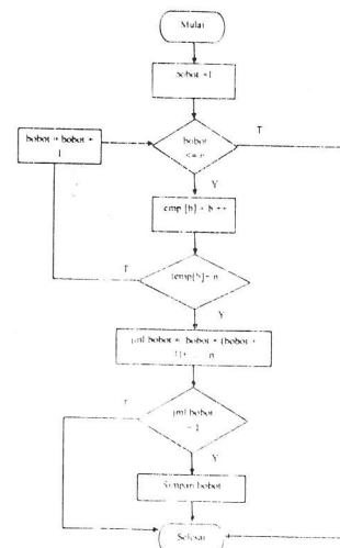
Gambar 7. Standarisasi Bobot Sesuai dengan KPI
