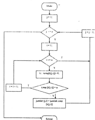
Gambar 3. Penjumlahan skala perbandingan setiap kriteria perbaris.
