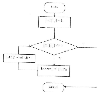
Gambar 6. Pembagian Jumlah Kriteria Perkolom dengan Banyaknya Kriteria
