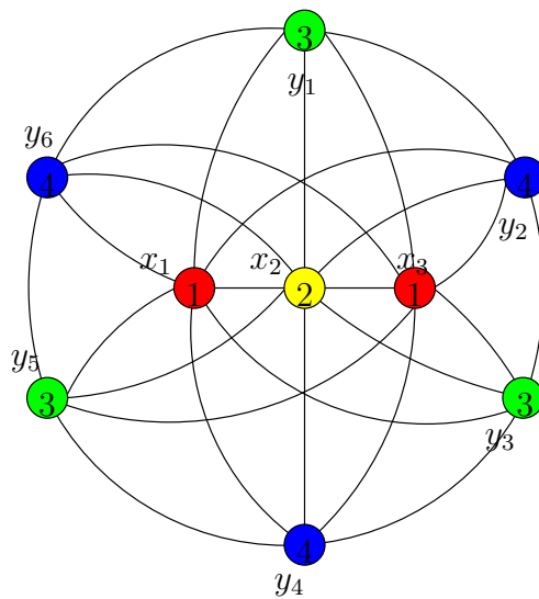
Figure 1: Contoh pewarnaan titik (P_n + C_m) untuk m genap
