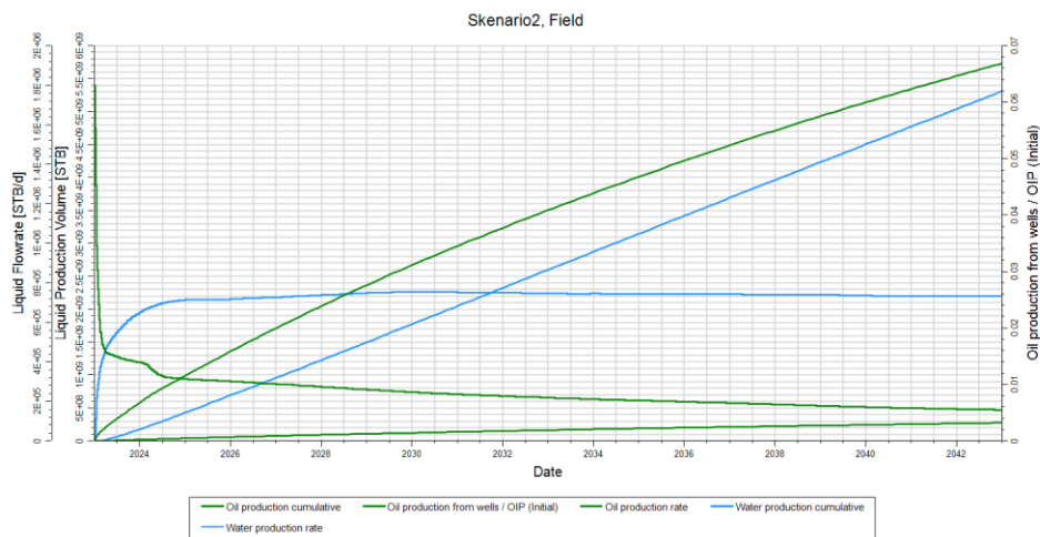
Gambar 4.20 Grafik Produksi Skenario Pengembangan Kedua
