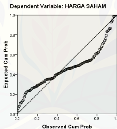
Gambar 2 Hasil Uji Normalitas dengan probability plot
