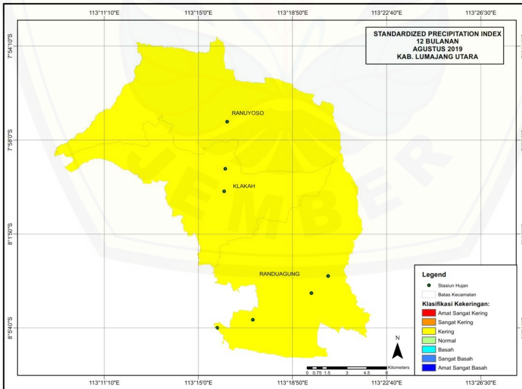
GAMBAR 11. Kekeringan tahun 2019
