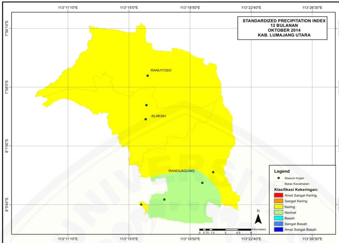
GAMBAR 6. Kekeringan tahun 2014
