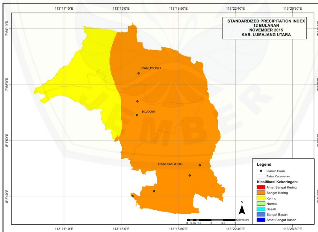
GAMBAR 7. Kekeringan tahun 2015
