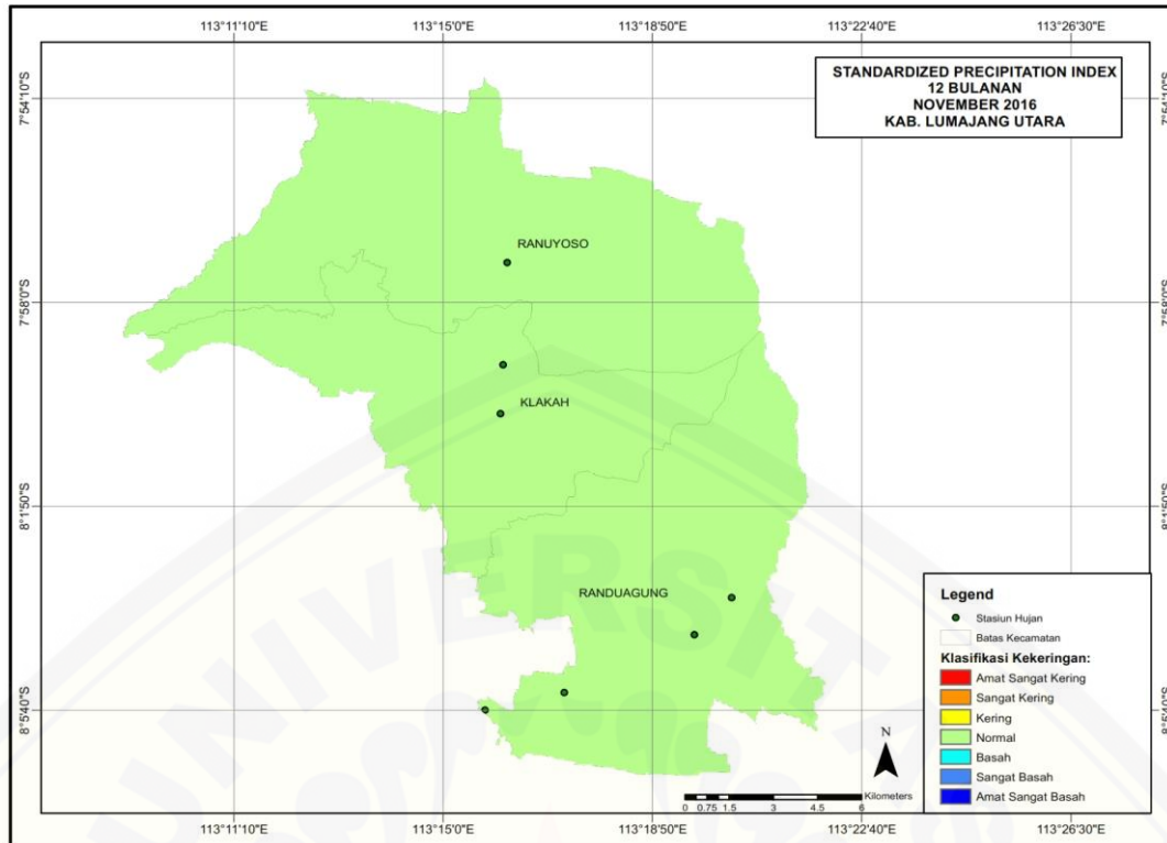
GAMBAR 8. Kekeringan tahun 2016
