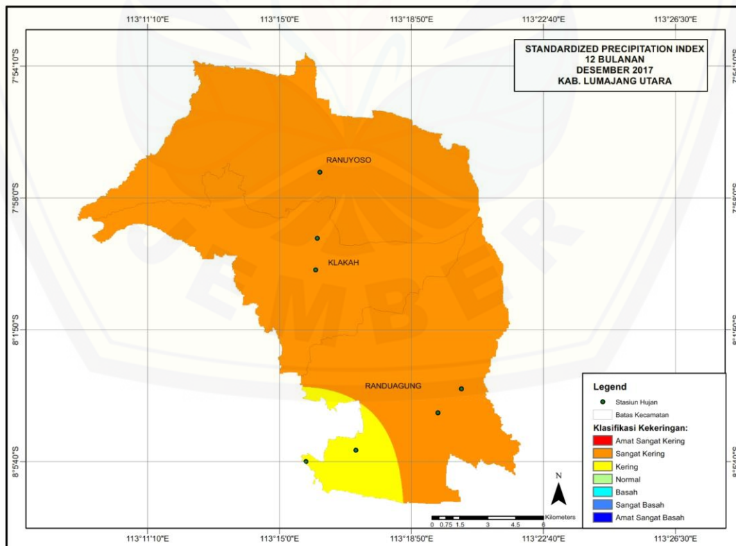
GAMBAR 9. Kekeringan tahun 2017
