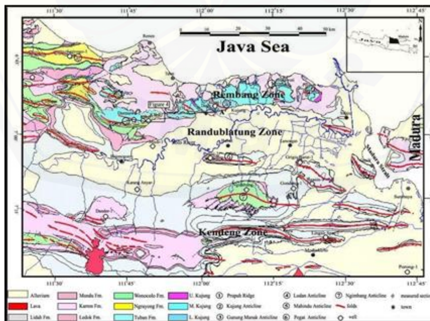
Gambar 1. Geologi Regional Jawa Timur Utara
