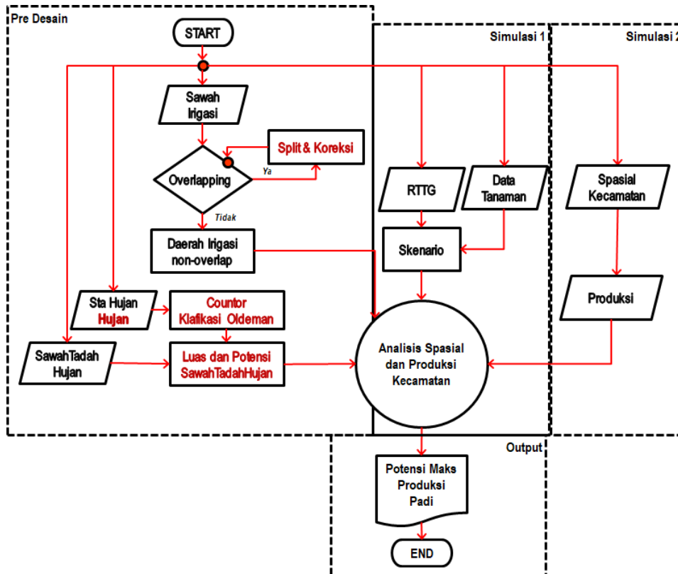
Gambar1. Diagram Metodologi
